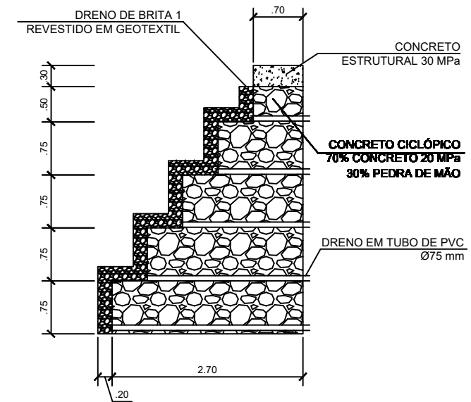
CORTE AA s./ESC.
