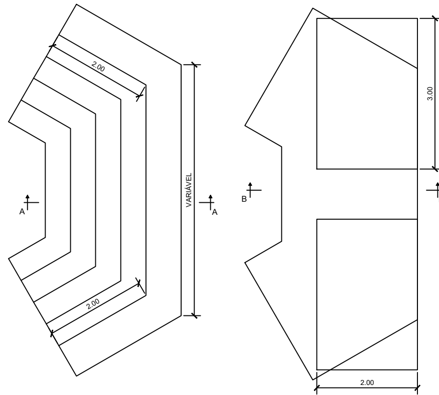
FUNDAÇÃO s./ESC.
