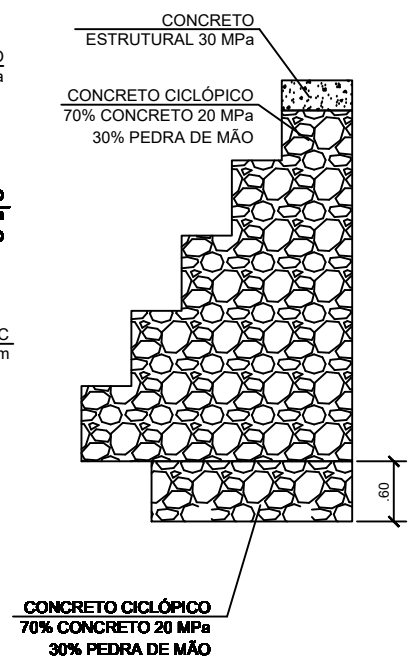
CORTE BB s./ESC.
