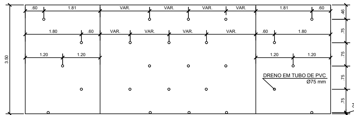
DRENO VISTA FRONTAL s./ESC.
